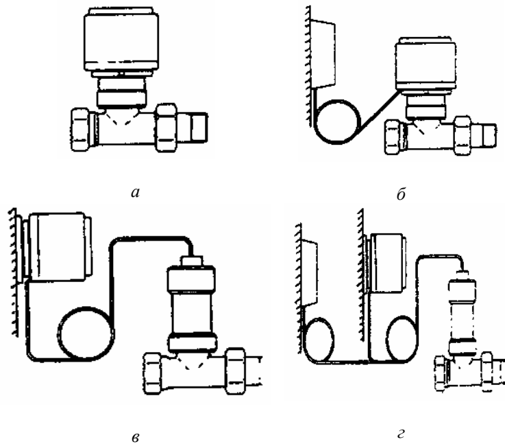
a — терморегулятор со встроенным регулятором температуры и датчиком; б — терморегулятор со встроенным регулятором температуры и дистанционным датчиком; в — терморегулятор с дистанционным датчиком, который объединен с регулятором температуры; г — терморегулятор с дистанционным датчиком и отдельно расположенным регулятором температуры
